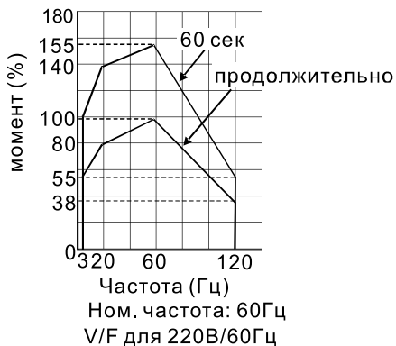
Асинхронный двигатель
