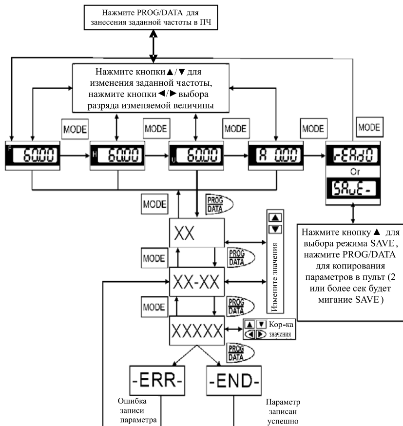
Алгоритм работы пульта VFD-PU06
