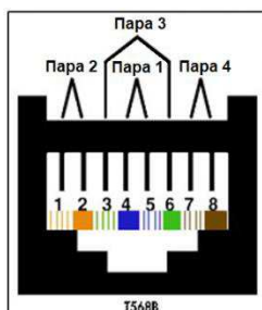
Рис. 3-19 Стандартный T568B
